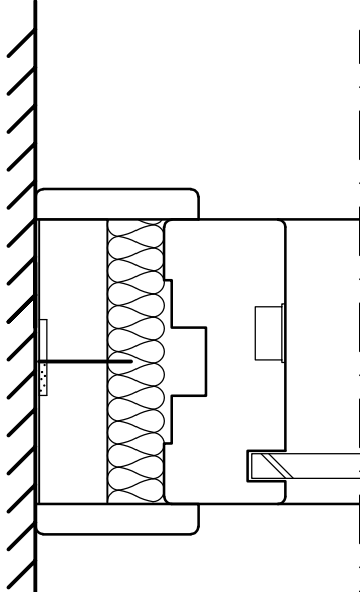
DETALJ 01.
